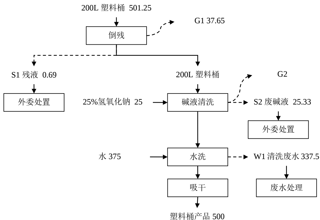
图 3.8-1 200L 塑料桶清洗工艺物料平衡图
