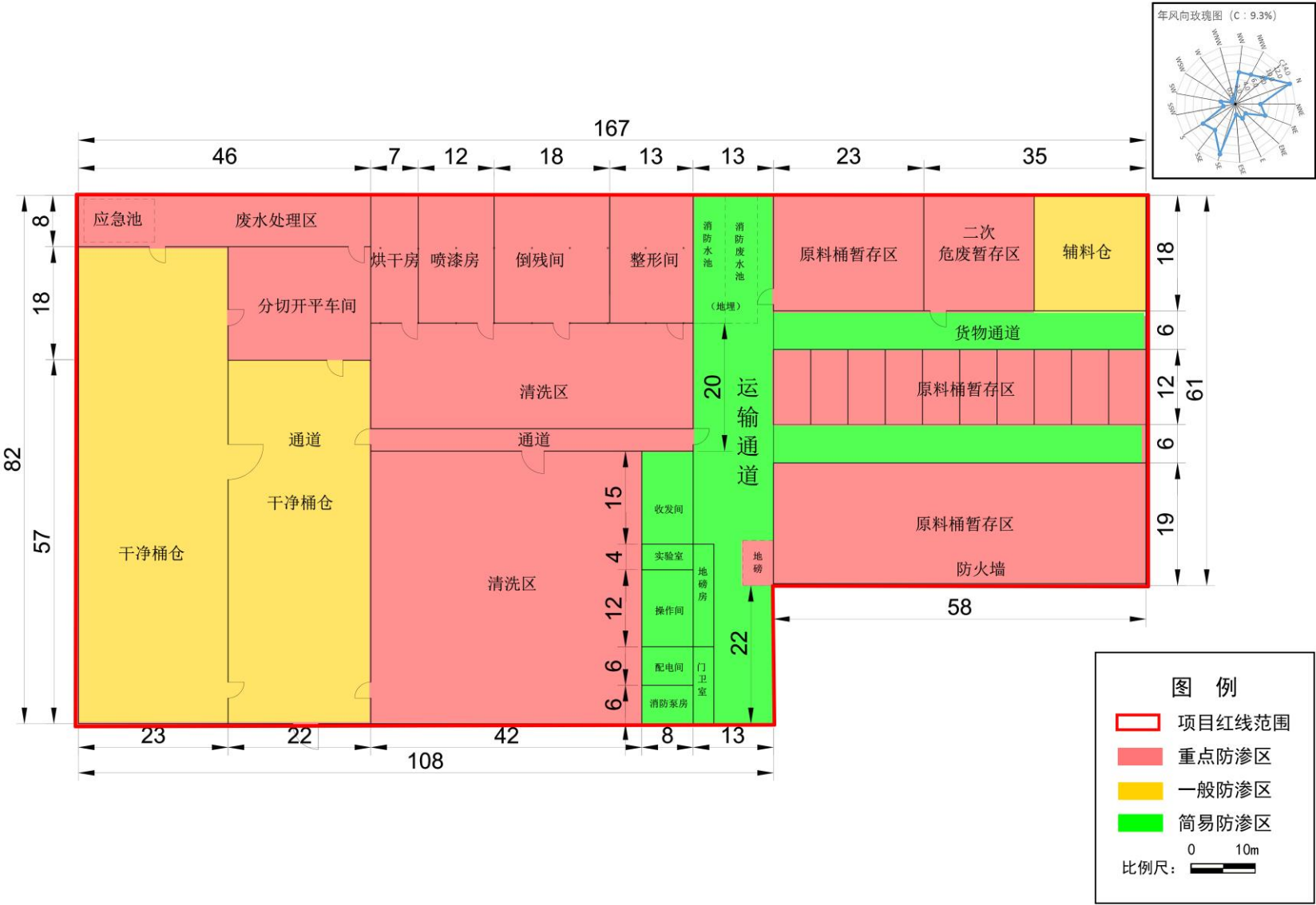
图 6.5-1 项目地下水分区防治示意图
