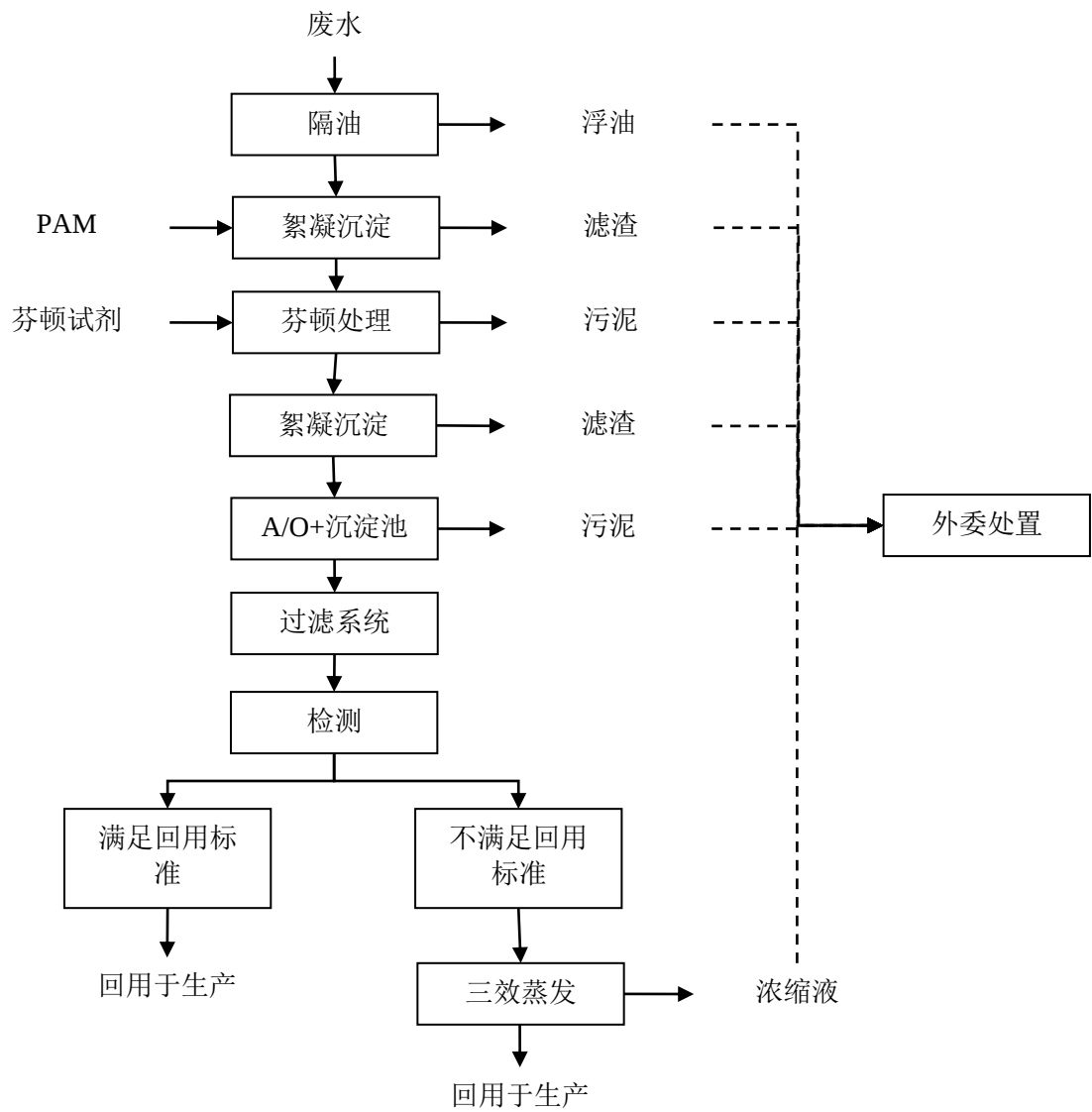
图3.9-1 生产废水处理工艺流程图
